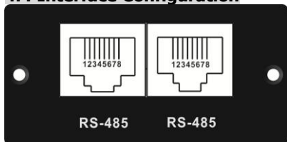
RS-485 Pin Configuration
